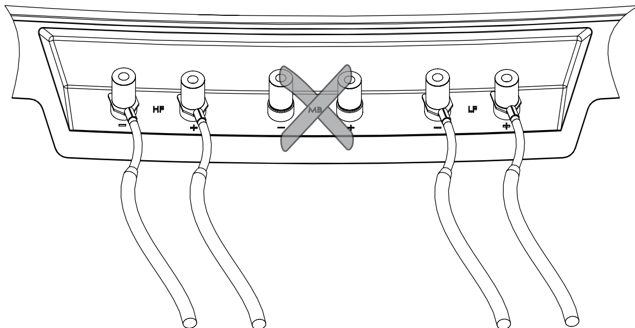
Terminales traseros
