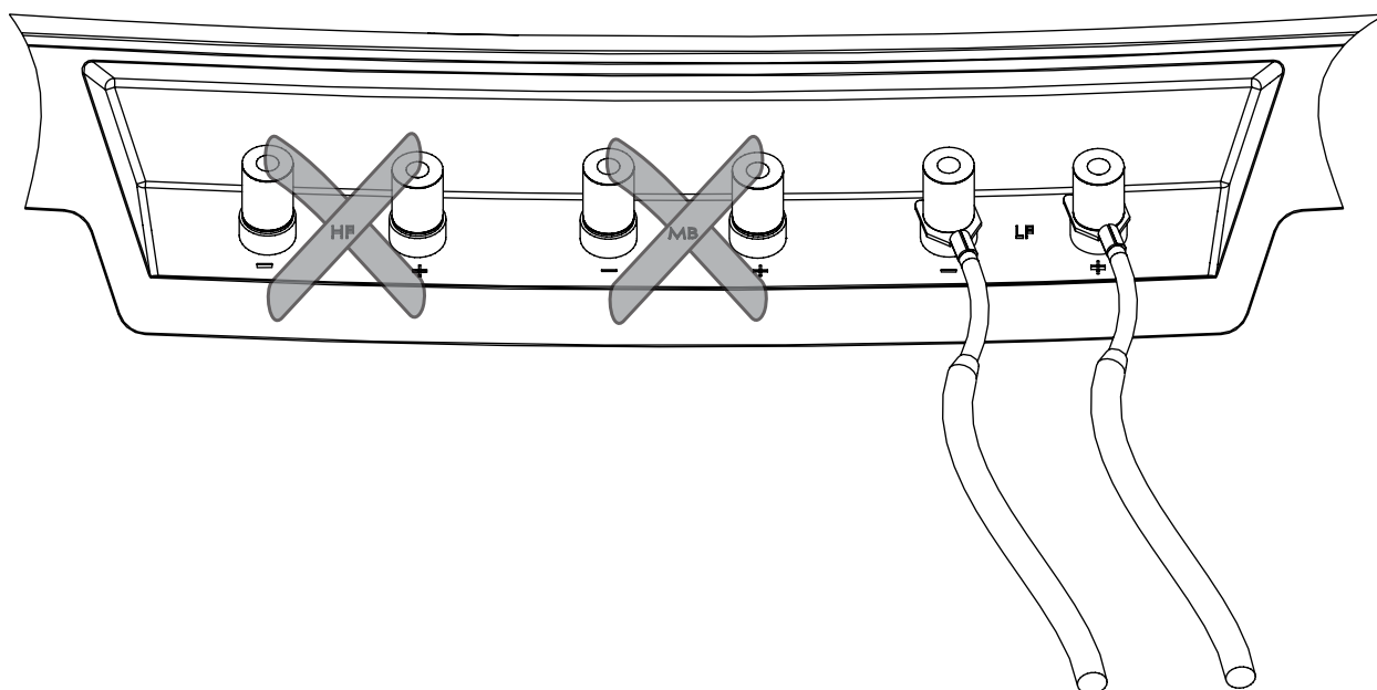
Terminais Traseiros
